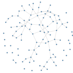
Erdős-Rényi
