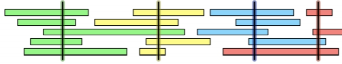
Figura 2: Exemple d'un conjunt d'interval·ls interceptats per 4 punts (representats com a segments verticals).
